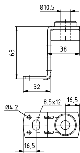
Luchtkanaal-dubbelhoek Type I
