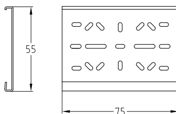
StaboFix® Fixeerplaat
