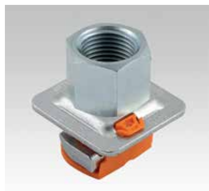
Uitvoering M16 + R \frac{1}{2} "
