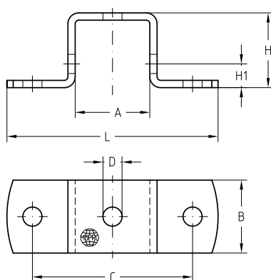
Voor profielen 28/30
