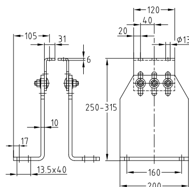
Zware uitvoering, grotere afstand tot het bouwlichaam
