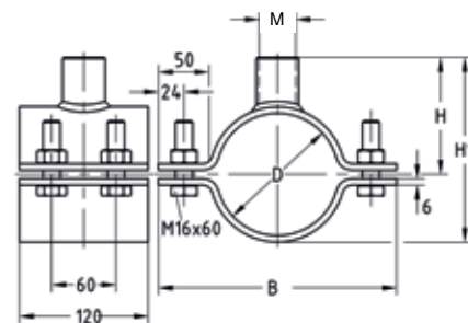
Vastpuntbeugel 120 x 6
