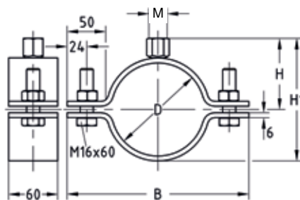
Vastpuntbeugel 60 x 6
