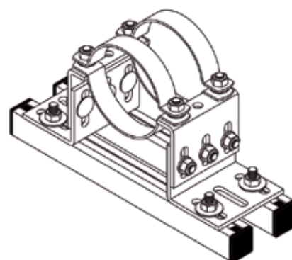
Vrij verschuifbare opstelling
