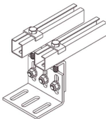
In hoogte verstelbare onderconstructie voor vastpunten en glijbevestigingen
