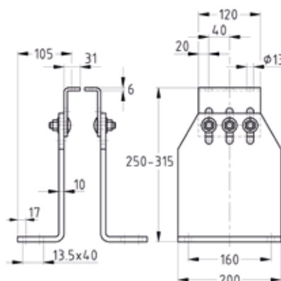
Zware uitvoering, grotere afstand tot het bouwlichaam
