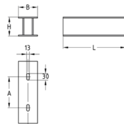
Voor profiel Q80, Q150, schets (origineel kan afwijken)
