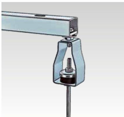
Geluiddempingsophanger M10
